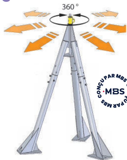
TRIPODE ACIER GALVANISÉ Épaisseur 5 mm - Ø 139 mm
