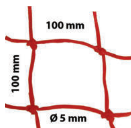
NF S 52106 S1 POLYÉTHYLÈNE HD Rouge avec ralingue
